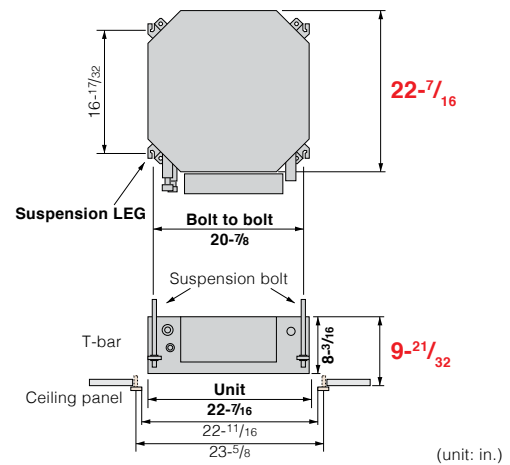
■ NTXCKS12A112A*
