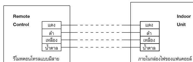
รีโมทคอนโทรลแบบมีสาย
