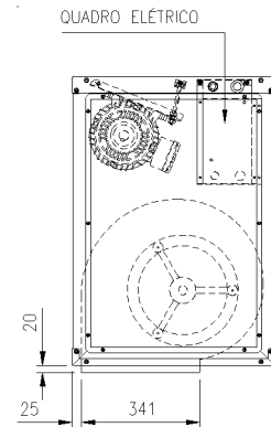
Fig. 07c - Descarga Piso
