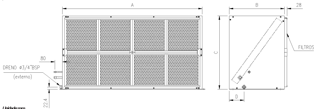
Fig. 14 - Dimensional Módulo Serpentina 350 a 500
