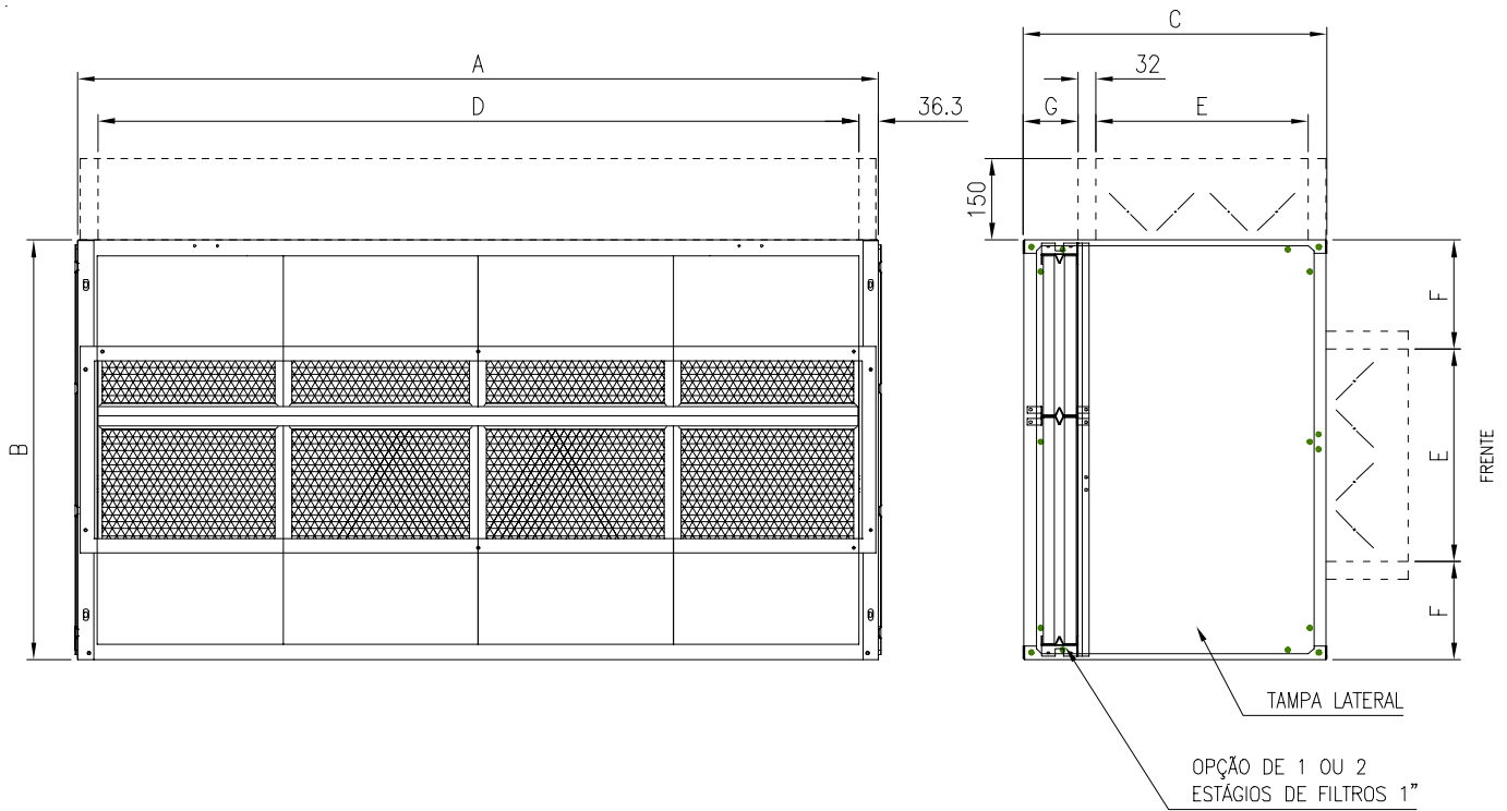
Fig. 15 - Dimensional Módulo Caixa de Mistura
